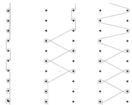
經編織圖 Warp Transmitting Pattern
