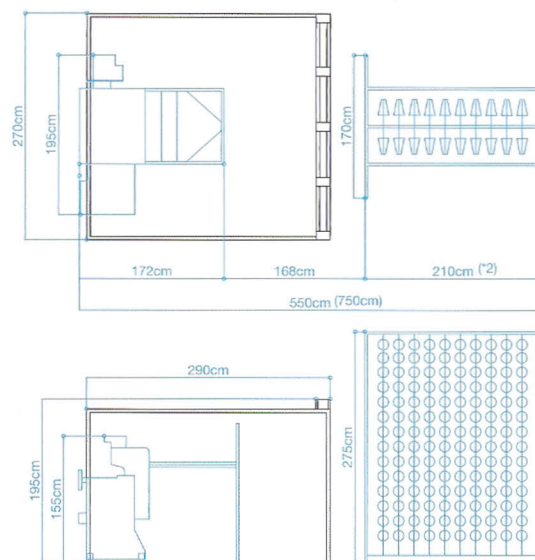
場地規劃 Site Plan
